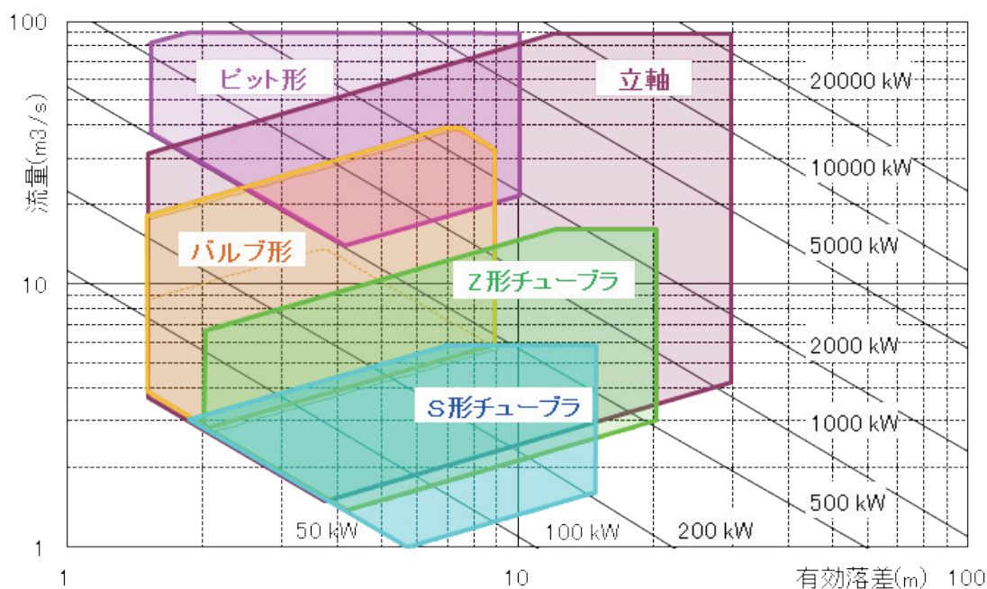
図. カプラン水車の選定表
